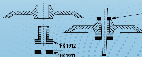
Stop-ring integrated with the shaft/ mit Schaft integriert/intégré à l'arbre/ integrato con l'albero
